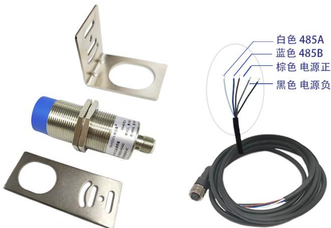
图3 RS-485 接口款
