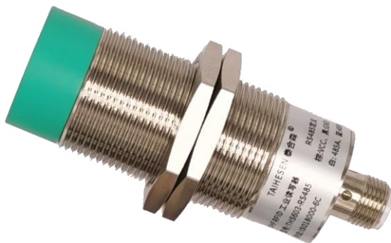
图1 读写器外形
